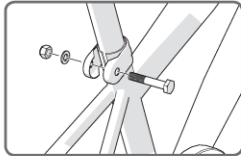
ALTİKÖŞE BAŞLI CİVATALI SELE BAĞLANTISI
