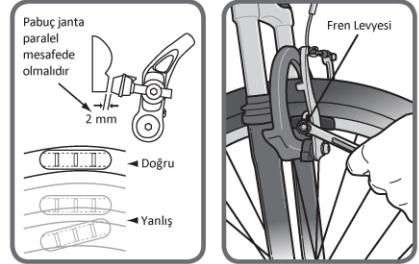
Fren Pabuç Ayarı
